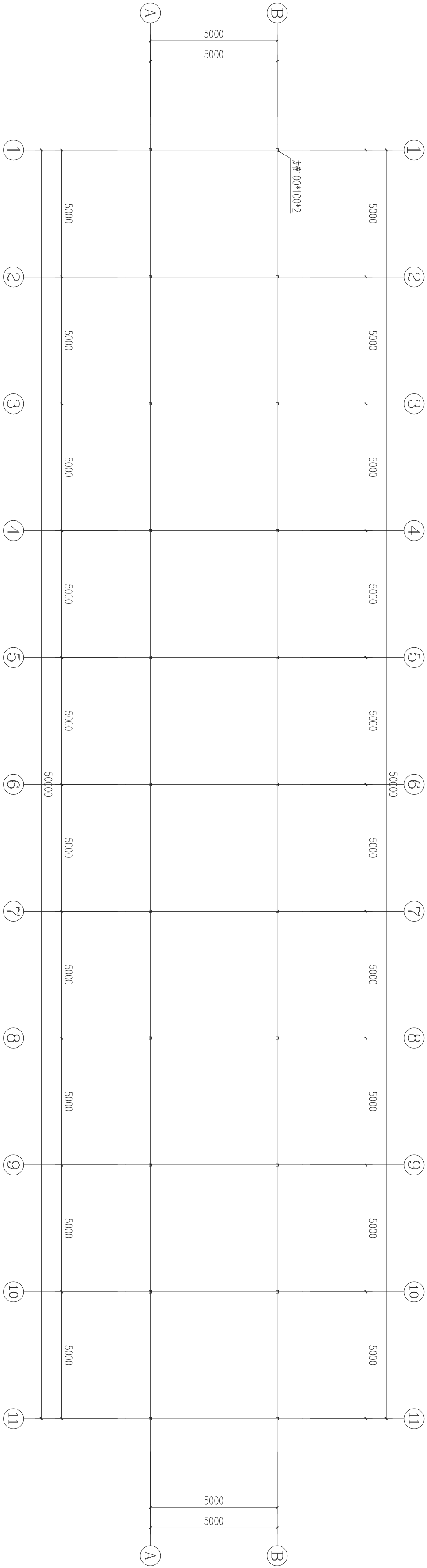
一层平面图 1:150
